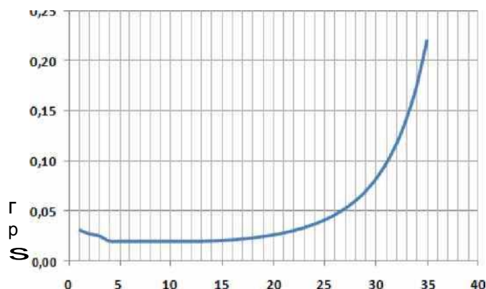
Рисунок 18. Интенсивность отказов в зависимости от срока эксплуатации участка тепловой сети
