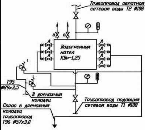
Принципиальная схема обвязки котла КВр-1,25
