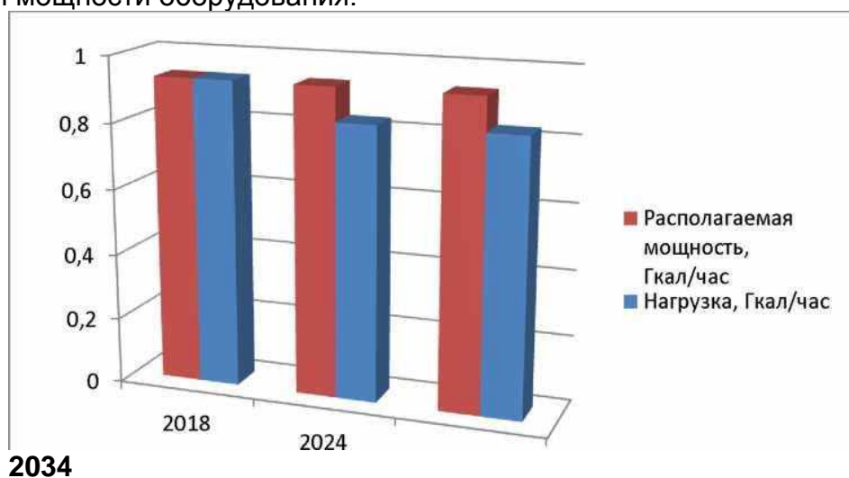
Рисунок 14. Диаграмма изменения нагрузки по отношению к располагаемой мощности оборудования
