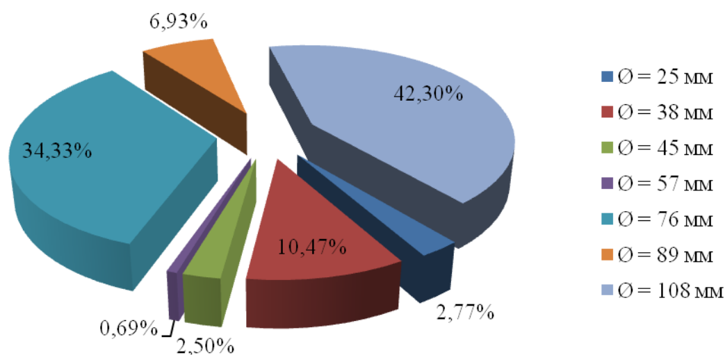
Рисунок 2.3.2.2 – Доли протяжённости участков трубопроводов тепловых сетей котельных МУП ТС «Ремовский» различных диаметров
