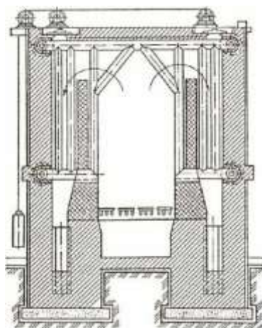
Рис.3. Секция котла НР-18 из гнутых труб.1,2 - вертикальные стальные трубы ф - 89 мм
