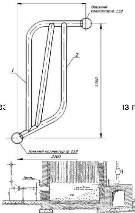
Рис. 2. Продольный разрез котла НР-18
