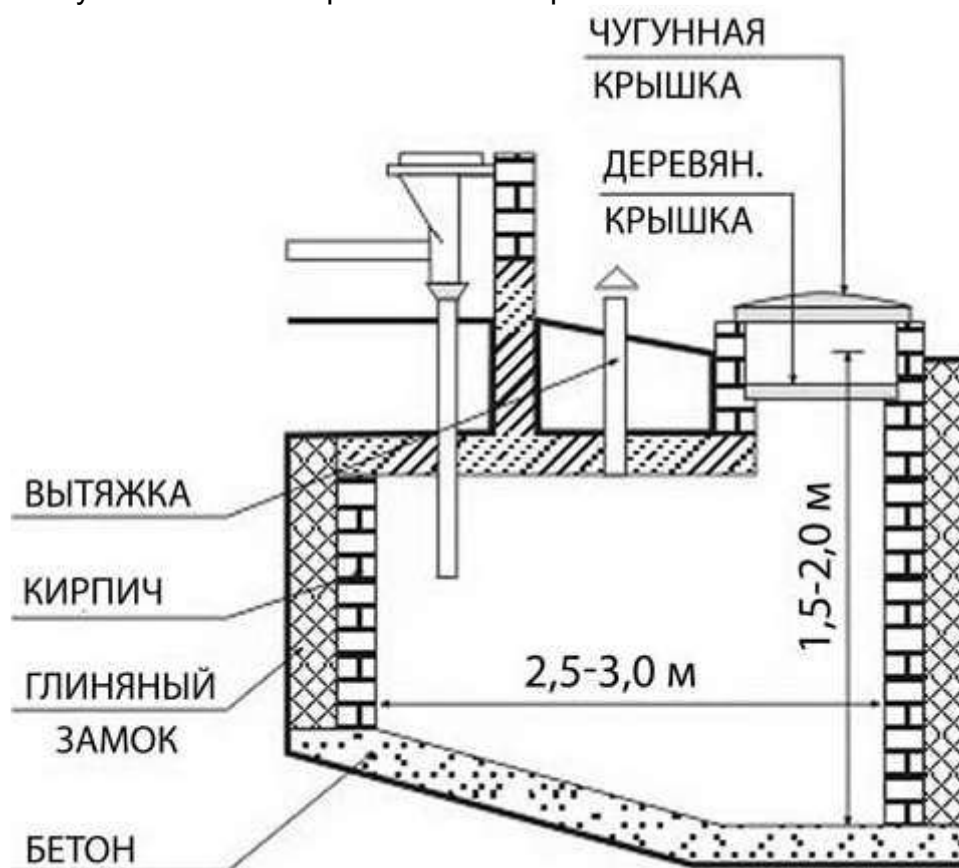
Рисунок 1 – Схема простейшей выгребной ямы из бетона
