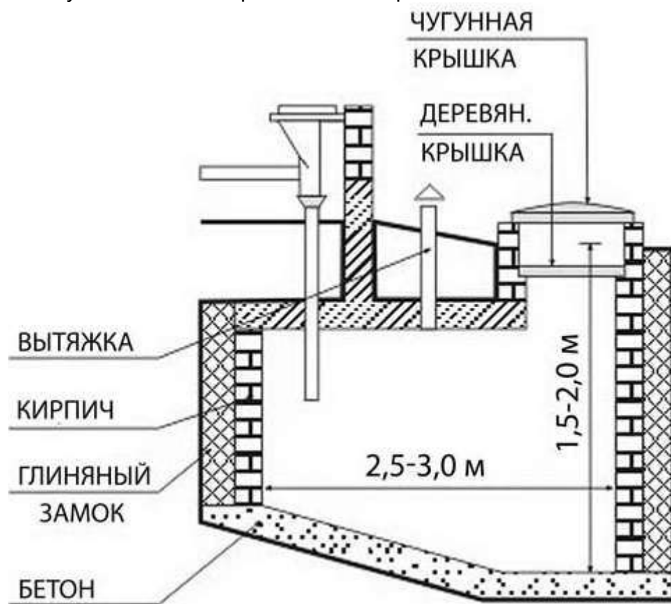
Рисунок 1 – Схема простейшей выгребной ямы из бетона
