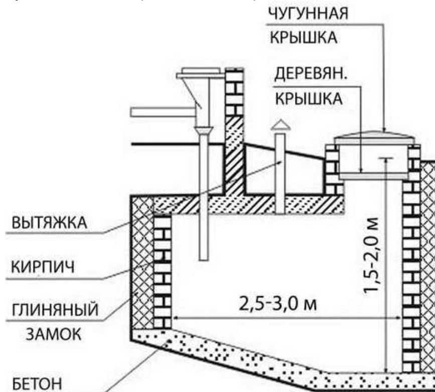
Рисунок 1 – Схема простейшей выгребной ямы из бетона
