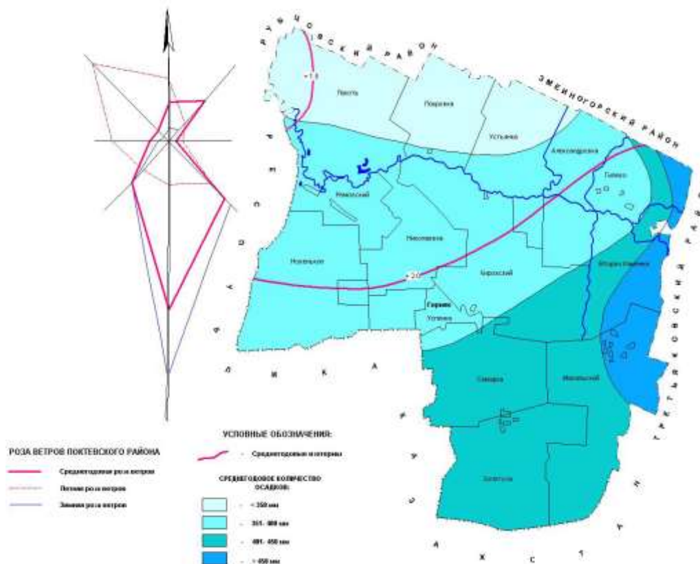
Рисунок 2 – Схема распределения среднегодовых температур и атмосферных
